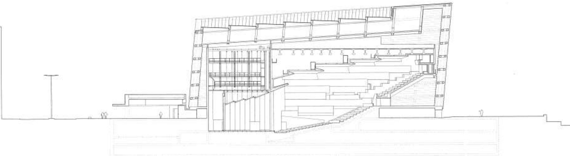
Sección Auditorio / Auditorium section
