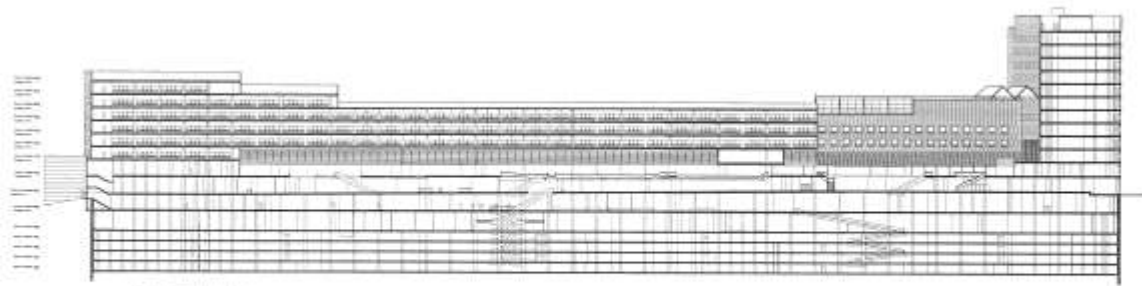
Wohngebäude Längsschnitt
