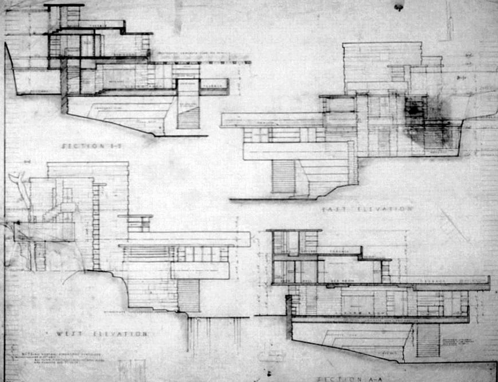
SECTION A-A
