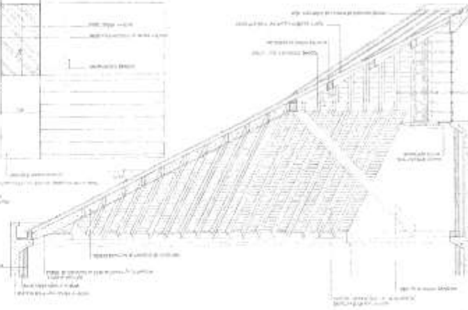
DETALLE DE LA CUBIERTA 3-3
