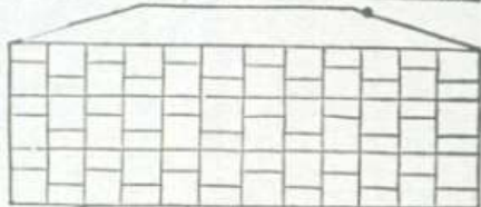
incertum
