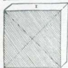
tetradoron didoron
