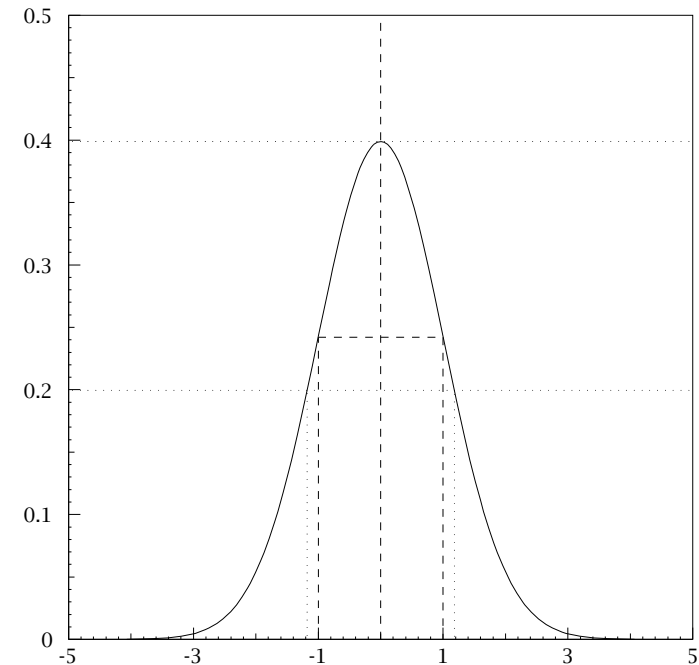
FIGURA 8c - L'andamento della funzione N(x; 0, 1) per la variabile normale standardizzata (ossia con media 0 e varianza 1).
