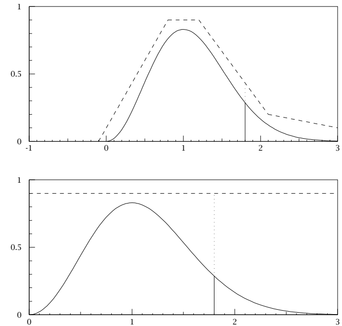
FIGURA 8b - La scelta di un numero a caso con distribuzione prefissata mediante tecniche numeriche (la densità di probabilità è la stessa della figura 4d); la funzione maggiorante è una spezzata (superiormente) o la retta y = 0.9 (inferiormente).
