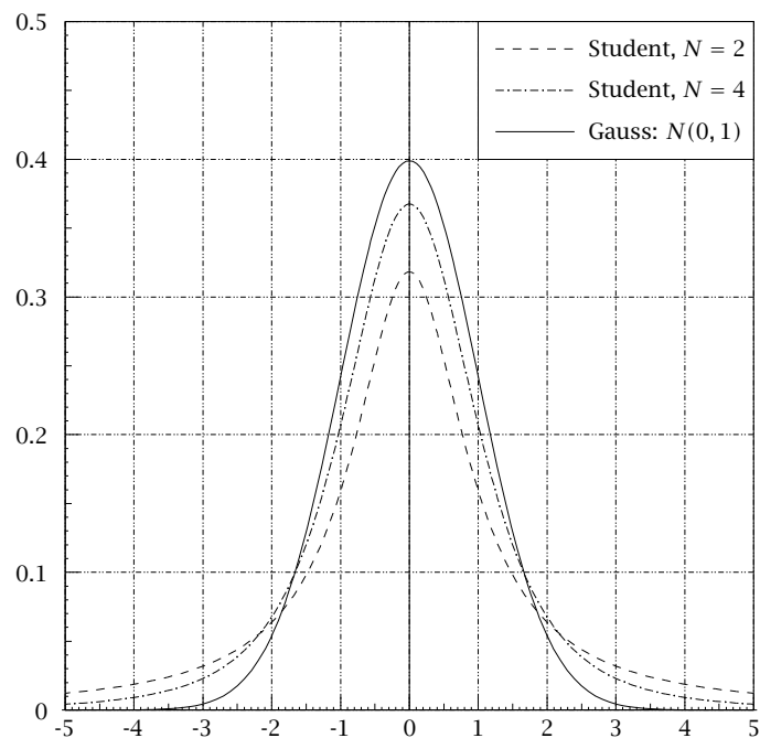
FIGURA 12e - La distribuzione di Student per N = 2 ed N = 4 , confrontata con la funzione normale.
