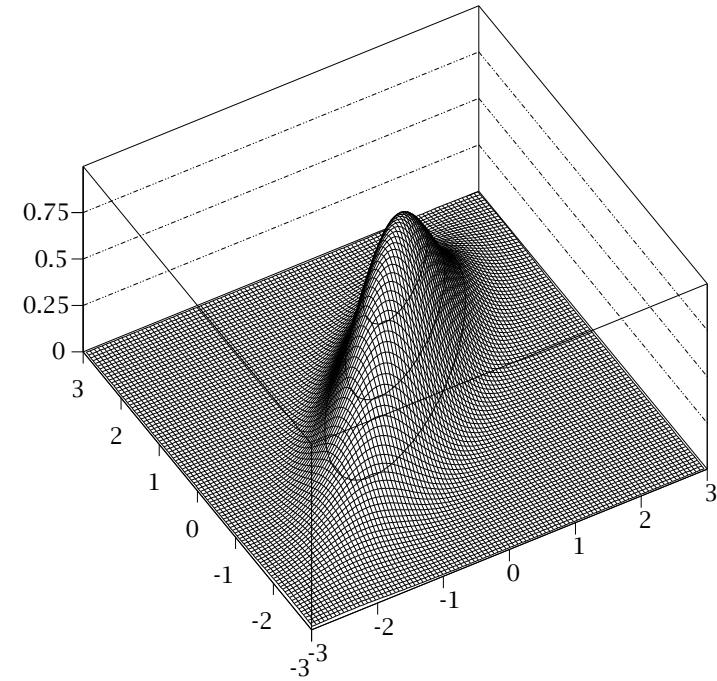
FIGURA 8i - La funzione normale in due dimensioni, nel piano \{u, v\} delle variabili standardizzate e per un coefficiente di correlazione r = 0.8 .
