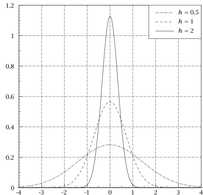
FIGURA 9a - La funzione di Gauss per tre diversi valori di h .
