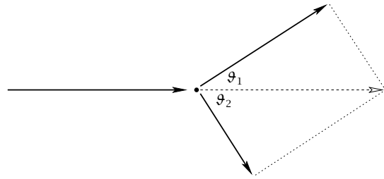
FIGURA 12d - Urto elastico protone-protone.
