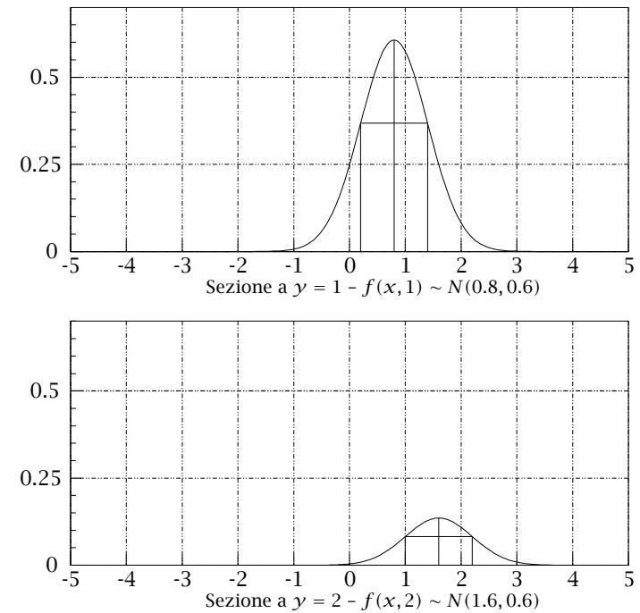
FIGURA 8k - Le sezioni della figura 8i con due piani di equazione y = 1 e y = 2 rispettivamente: ovvero (a parte la normalizzazione) le densità di probabilità condizionate \pi(x|y = 1) e \pi(x|y = 2) .
