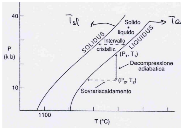
Fig. 2.2 - Variazione della temperatura di fusione ( T_{st} ) e di inizio cristallizzazione ( T_{iq} ) in funzione della pressione per un magma basaltico anidro. Per una data pressione la differenza ( T_{iq}-T_{st} ) rappresenta l'intervallo di cristallizzazione per quella profondità. Un magma nella posizione 1 a ( P_1, T_1 ), se risale adiabaticamente, diviene sovrariscaldato.
