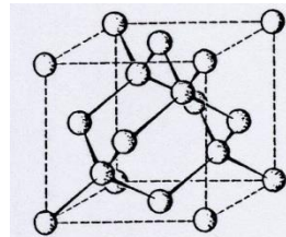
Fig. 12.2 Struttura del diamante. Ciascun atomo di carbonio ne coordina tetraedricamente altri quattro, cui è collegato da legami sp^3 ; i collegamenti vertice a vertice fra un numero indefinito di tetraedri determinano il formarsi di un'unica macromolecola grande quanto tutto il cristallo.
