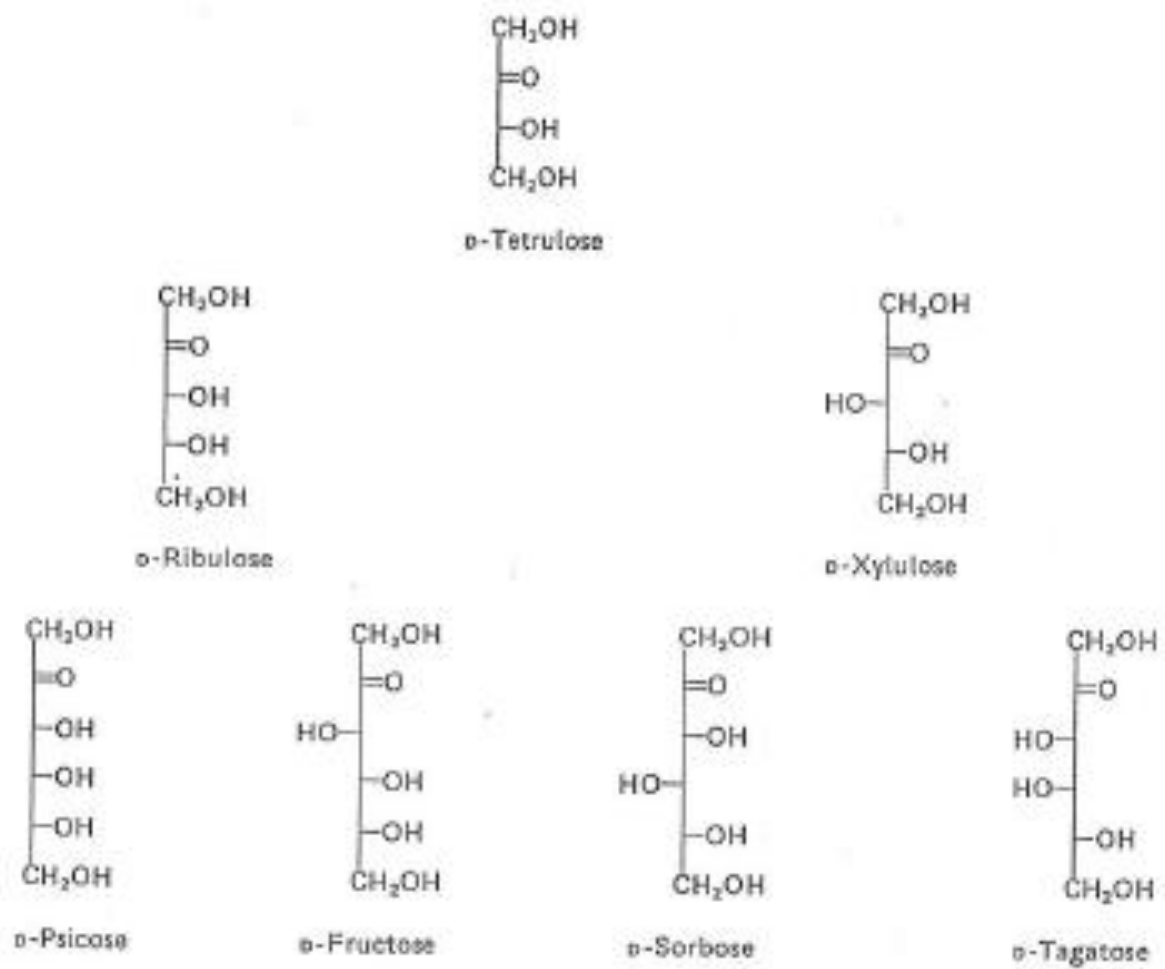
Fig. 4.2. D-Ketoses in Fischer projection
