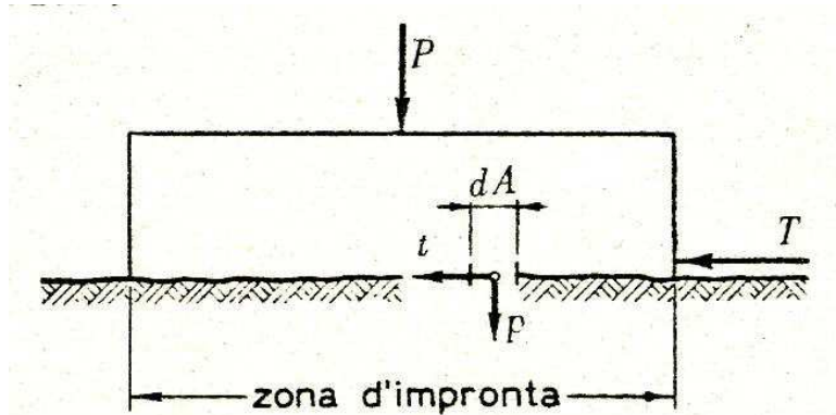
Fig. 42. - Forze unitarie normali e tangenziali fra due superfici piane a contatto
