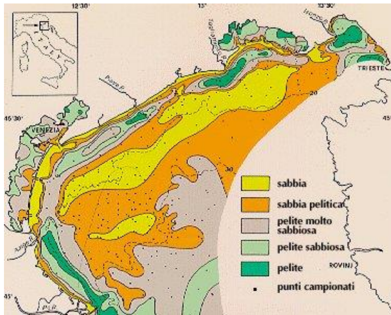
Carta sedimentologica dell'Alto Adriatico secondo la classificazione di Nota
