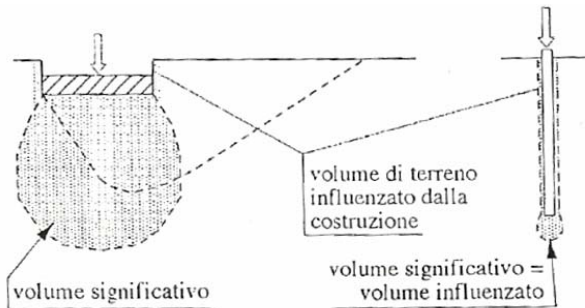
Figura 2. Volume significativo e volume di terreno influenzato dalla costruzione per una fondazione diretta e per un palo.
