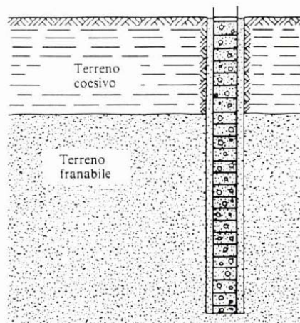
(d) Il palo a costruzione completata.
