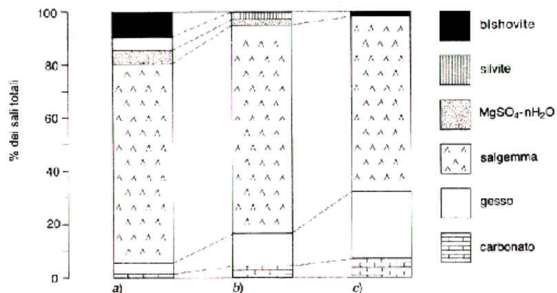
Fig. 6.5 - Abbondanza relativa dei principali sali. (a) precipitati in condizioni sperimentali per evaporazione di acqua marina normale; (b) presenti nella successione permiana dello Zechstein ; (c) presenti mediamente nei depositi evaporitici. Si noti l'eccesso di carbonati e solfati nelle successioni fossili. (Borchert e Muir, 1964; Schmalz, 1969.)
