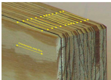
PIALLACCIO STRATIFICATO
