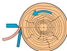
Piallaccio sfogliato
