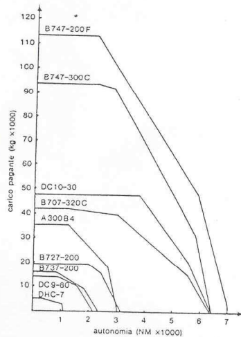
FIG. 1 - Curve «carico pagante (pay load) - autonomia (range)» di alcuni aeromobili commerciali (fonte: bibl., 2)
