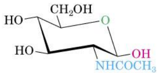
β-D-N-Acetilglucosamina (D-2-acetammino-2-deossiglucosio)
