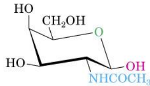
β-D-N-Acetilgalattosamina (D-2-acetammino-2-deossalattosio)
