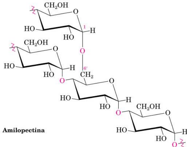
Amiloso, polimero del tipo 1,4'-O-( \alpha -D-glucopiranoside)
