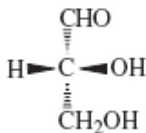
(R) -Gliceraldeide
