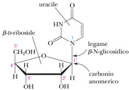
Uridina
