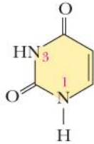
Uracile (U) RNA
