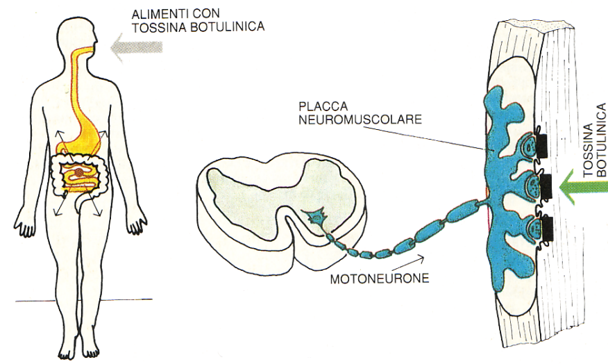
Schema del meccanismo genetico della paralisi spastica tipica del tetano ( in alto ) e quello della paralisi flaccida provocata dal botulismo. La tossina tetanica penetra a livello della giunzione neuromuscolare, ma, invece di agire a livello periferico, risale all'interno di vescicole l'assone del motoneurone. La tossina tetanica, scaricata nello spazio intersinaptico a livello del midollo spinale, penetra negli interneuroni inibitori bloccandone il rilascio di neurotrasmettitori. Ciò causa l'inibizione del meccanismo di bilanciamento della contrazione dei muscoli contrapposti che è controllato da questi interneuroni, dando origine a una paralisi spastica. Le neurotossine botuliniche penetrano anch'esse nel motoneurone a livello della giunzione dove inibiscono la liberazione di acetilcolina, bloccando la trasmissione dell'impulso nervoso al muscolo.
