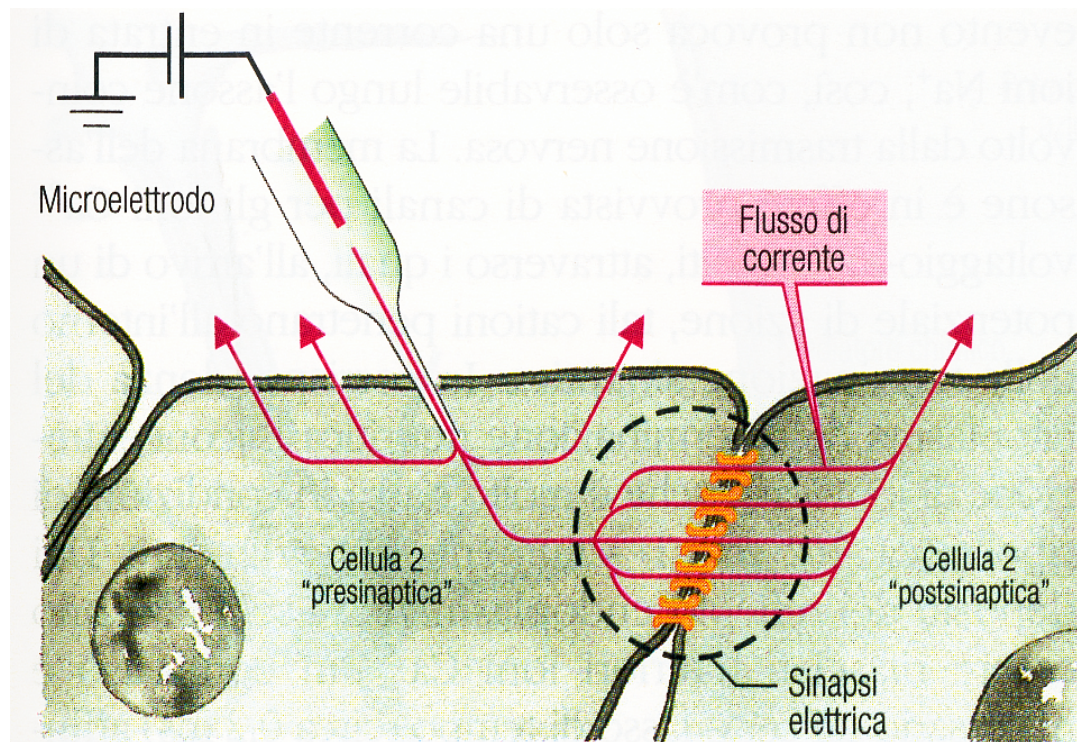
Figura 5.2 Quando, mediante un microelettrodo, viene applicata una corrente all'interno di una cellula coinvolta in una sinapsi elettrica, questa corrente si propaga direttamente attraverso il canale dei connessioni nell'adiacente "cellula postsinaptica" (→2). Allo stesso modo, a livello delle normali associazioni cellulari, una cellula presinaptica depolarizzata influenza la cellula a lei vicina.
