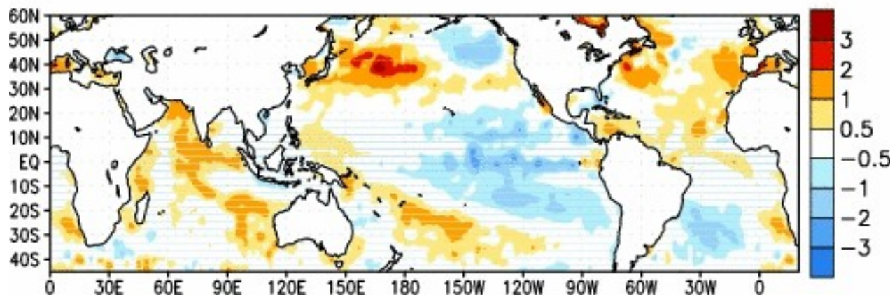
Medie settimanali della temperatura superficiale dell'oceano e anomalie rispetto alle medie climatiche (Reynolds and Smith 1995, J. Climate, 8, 1571-1583)) Anomalies (°C)
