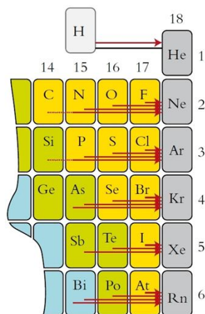
Figura 2A.4 Quando gli atomi dei non metalli acquistano elettroni dando origine agli anioni corrispondenti, si fermano nel momento in cui raggiungono la configurazione elettronica del gas nobile che segue.
