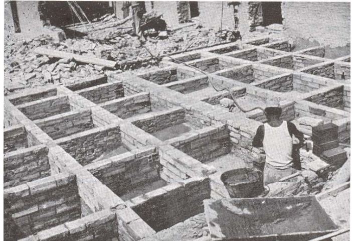
Frenelli su volta a crociera
