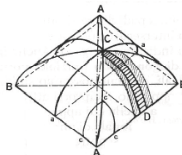
Volta a padiglione
