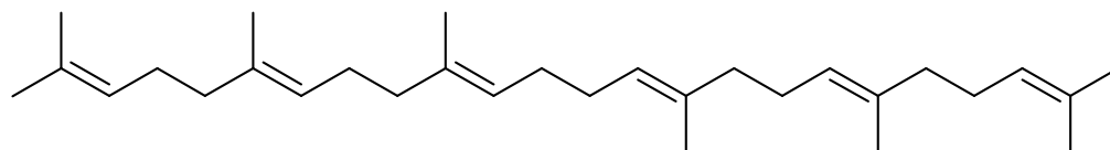
SQUALENE
