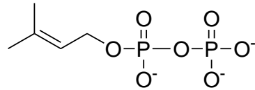
DMAPP dimetilallil difosfato
