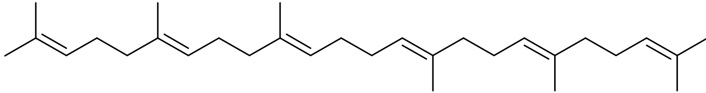
Squalene
