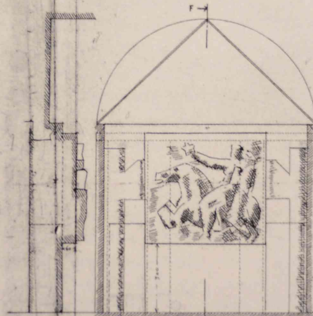
SEZIONE FF
