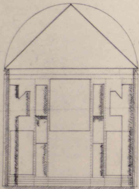
SEZIONE DD 1:50
