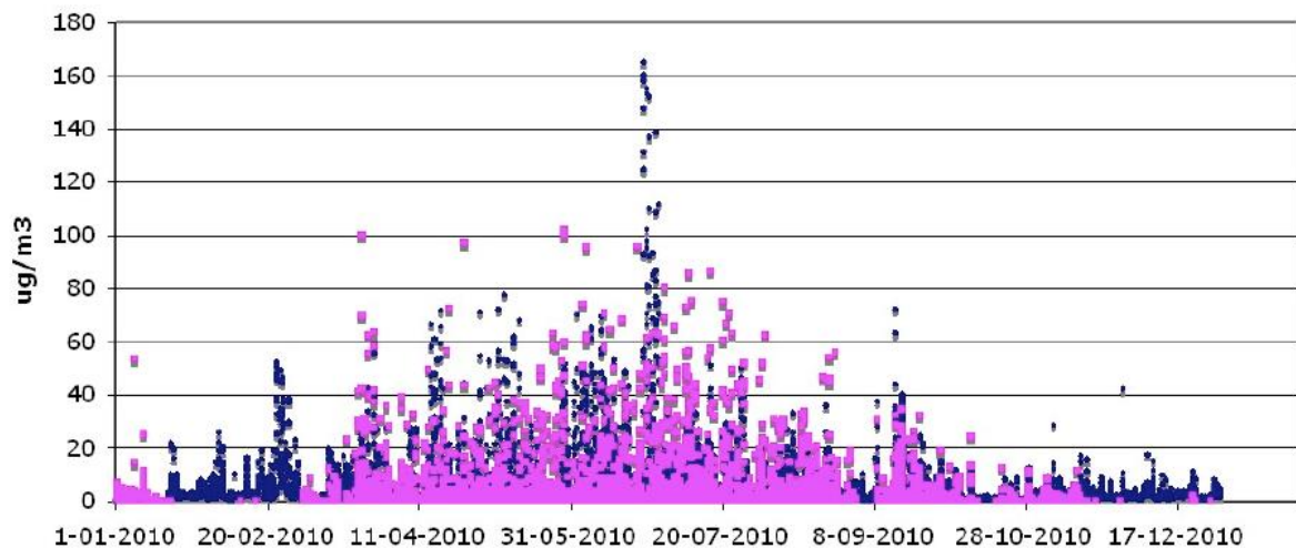
Concentrazioni orarie nel 2010
