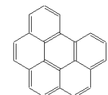
benzo[g,h,i]perilene
