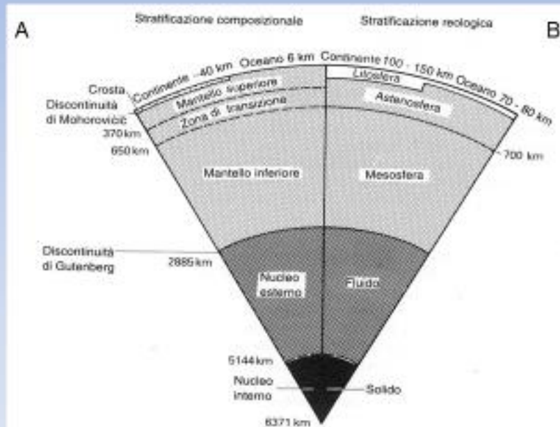
Figura 2.39 Confronto tra la stratificazione della Terra in base alla composizione e alla reologia .
