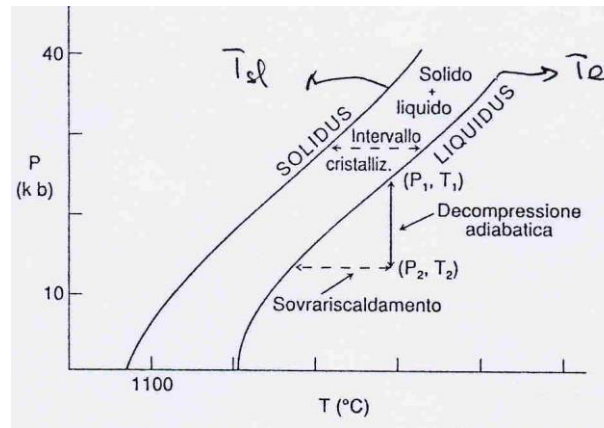
Fig. 2.2 - Variazione della temperatura di fusione ( T_q ) e di inizio cristallizzazione ( T_{iq} ) in funzione della pressione per un magma basaltico anidro. Per una data pressione la differenza ( T_{iq} - T_{st} ) rappresenta l'intervallo di cristallizzazione per quella profondità. Un magma nella posizione 1 a ( P_1, T_1 ), se risale adiabaticamente, diviene sovrarisaldato.
