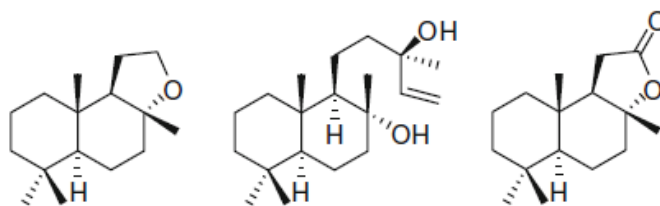
Figura 27. Strutture di (-)-Ambrox®, (-)-sclareolo e (+)-sclareolide. (Riadattato da ref 28 )
