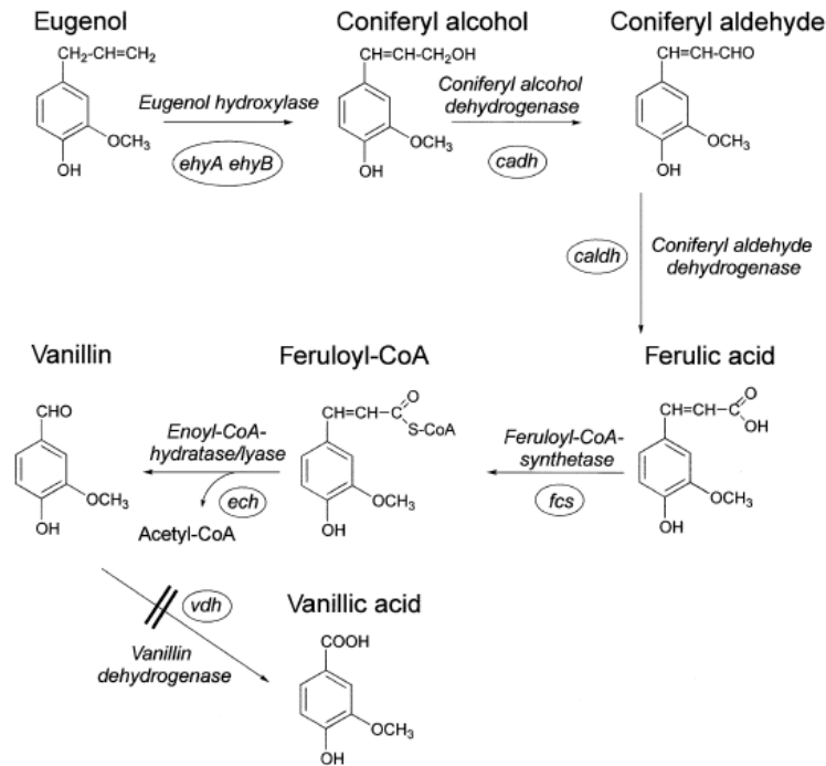
Figura 11. Sintesi della vanillina da eugenolo grazie a Pseudomonas sp. HR 199 geneticamente ingegnerizzato. (Riadattato da ref 24)
