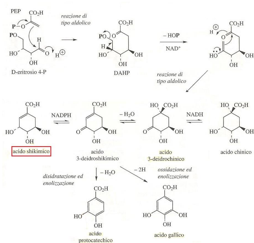
Figura 8. Reazioni iniziali della via dello shikimato. (Riadattato da ref 23 )
