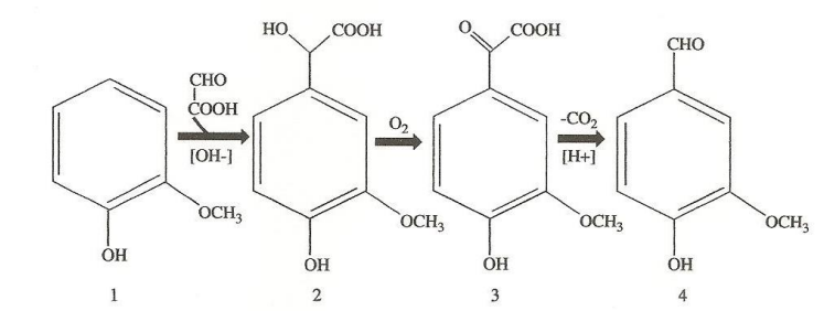
Figura 13. Sintesi della vanillina da guaiacolo. Guaiacolo (1), acido vanillilmandelico (2), acido 4-idrossi-3-metossifenilgliossilico (3) e vanillina (4). (Riadattato da ref 13)
