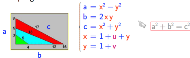
Terne pitagoriche
