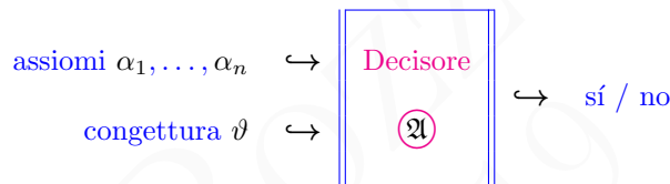
Figura 6: Schema di un ipotetico risolutore per l’ Entscheidungsproblem . Il “sì” direbbe che una dimostrazione di \vartheta esiste; il “no” che non esiste o addirittura che \vartheta è refutabile , nel senso che dagli assiomi discende l’esatto contrario, \neg\vartheta , di \vartheta . Da assiomi deboli potrebbe anche non discendere né \vartheta né \neg\vartheta e anche in questo caso la risposta del decisore sarebbe “no”.
