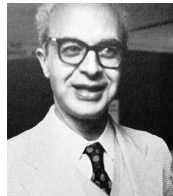
(Georg Kreisel, 1923–2015)
