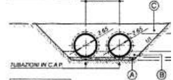
SEZIONE 7
