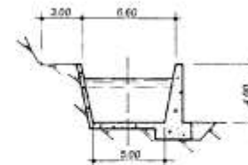
SEZIONE 4
