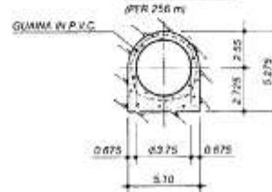
SEZIONE 3
