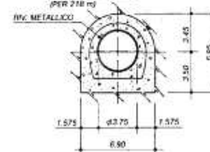
SEZIONE 4
