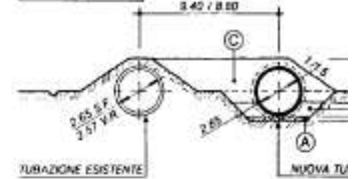
SEZIONE 7
