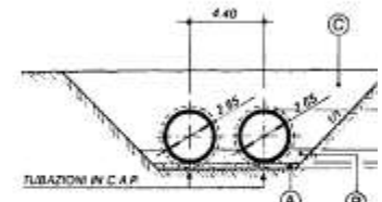
SEZIONE 6
