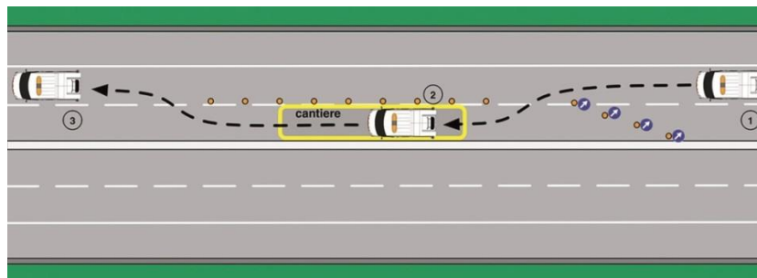
Figura 7 – Manovra di accesso e uscita dai cantieri in caso di chiusura della corsia di sorpasso
