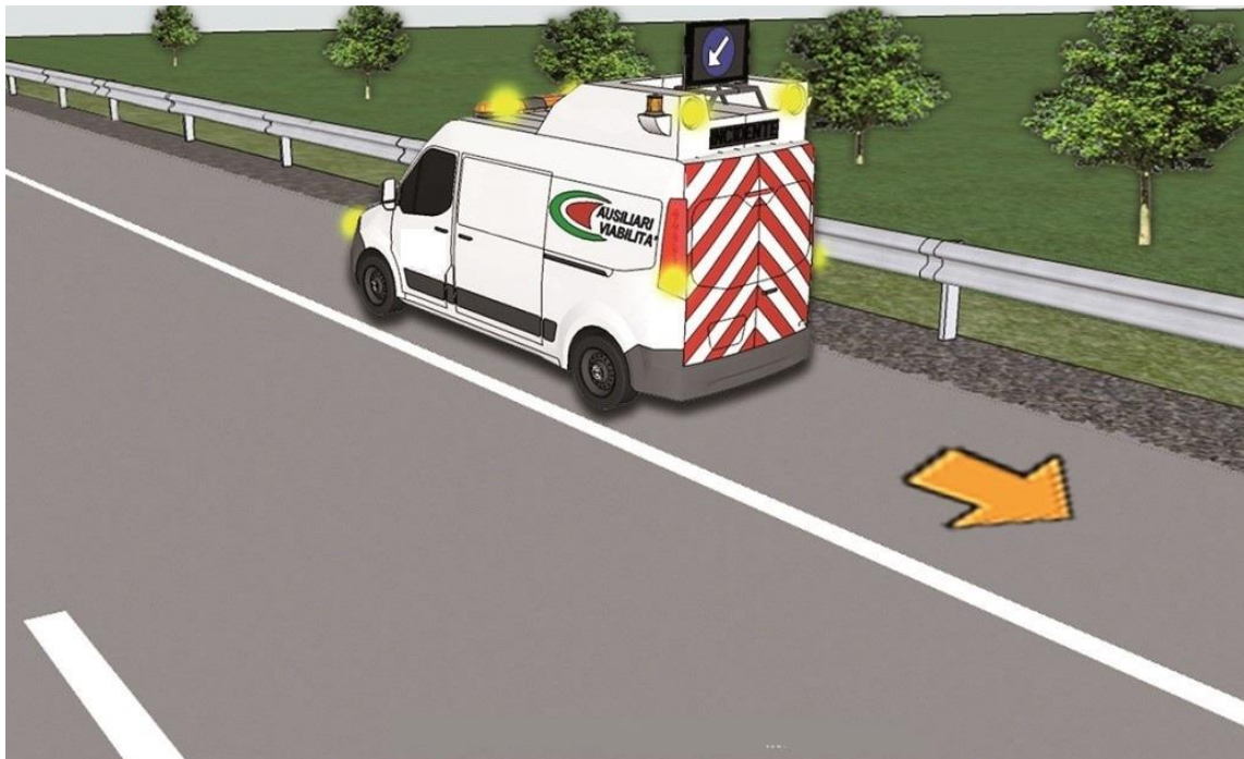
Figura 4 – Retromarcia in corsia di emergenza
