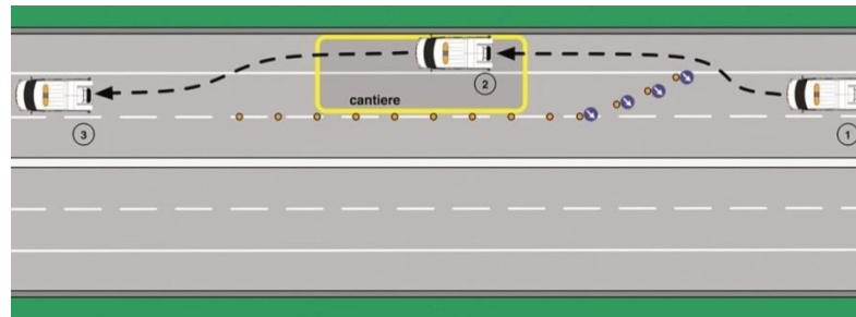
Figura 6 – Manovra di ingresso e uscita dai cantieri in caso di chiusura della prima corsia (corsia di marcia)
