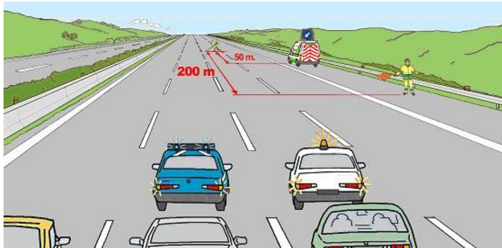
Figura 12 – Rallentamento controllato del traffico
