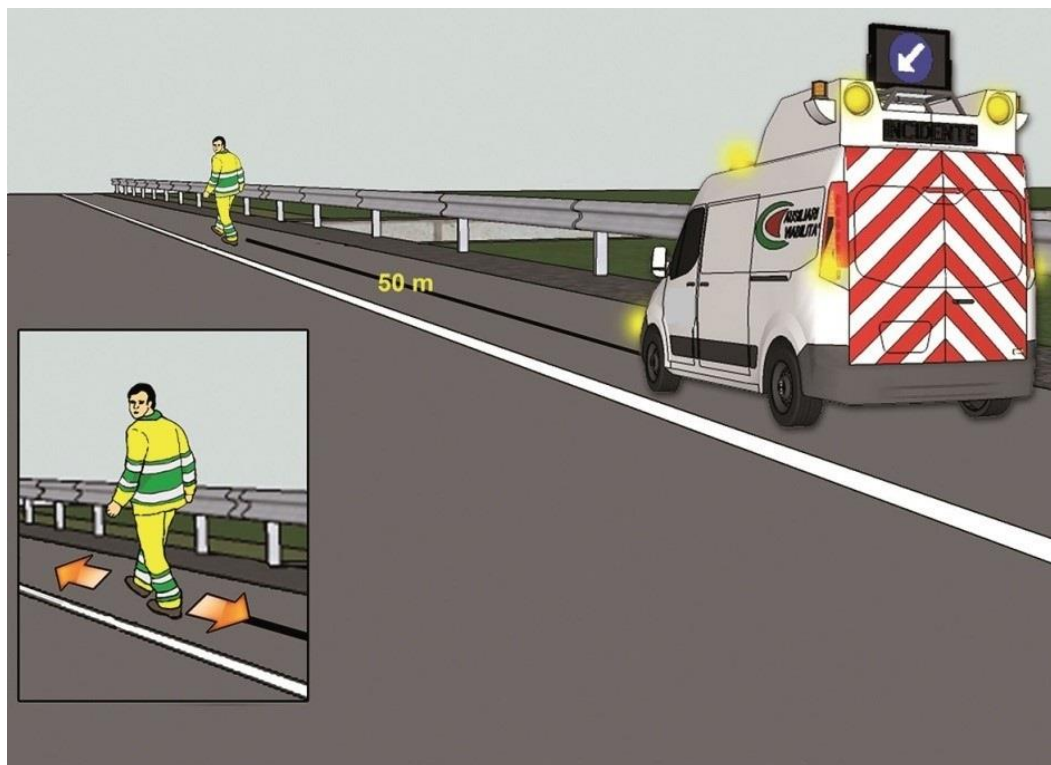
Figura 11 – Spostamento a piedi lungo la corsia d'emergenza
