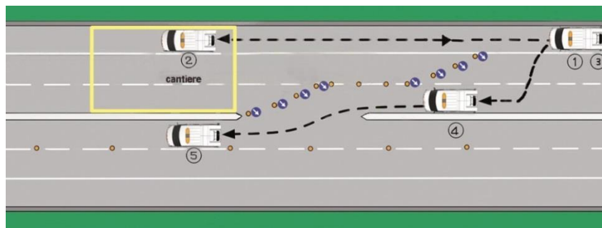
Figura 8 – Deviazione: Entrata ed uscita dal cantiere che occupa l'intera carreggiata transitabile
