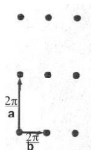
reticolo reciproco
