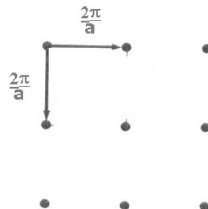
reticolo reciproco
