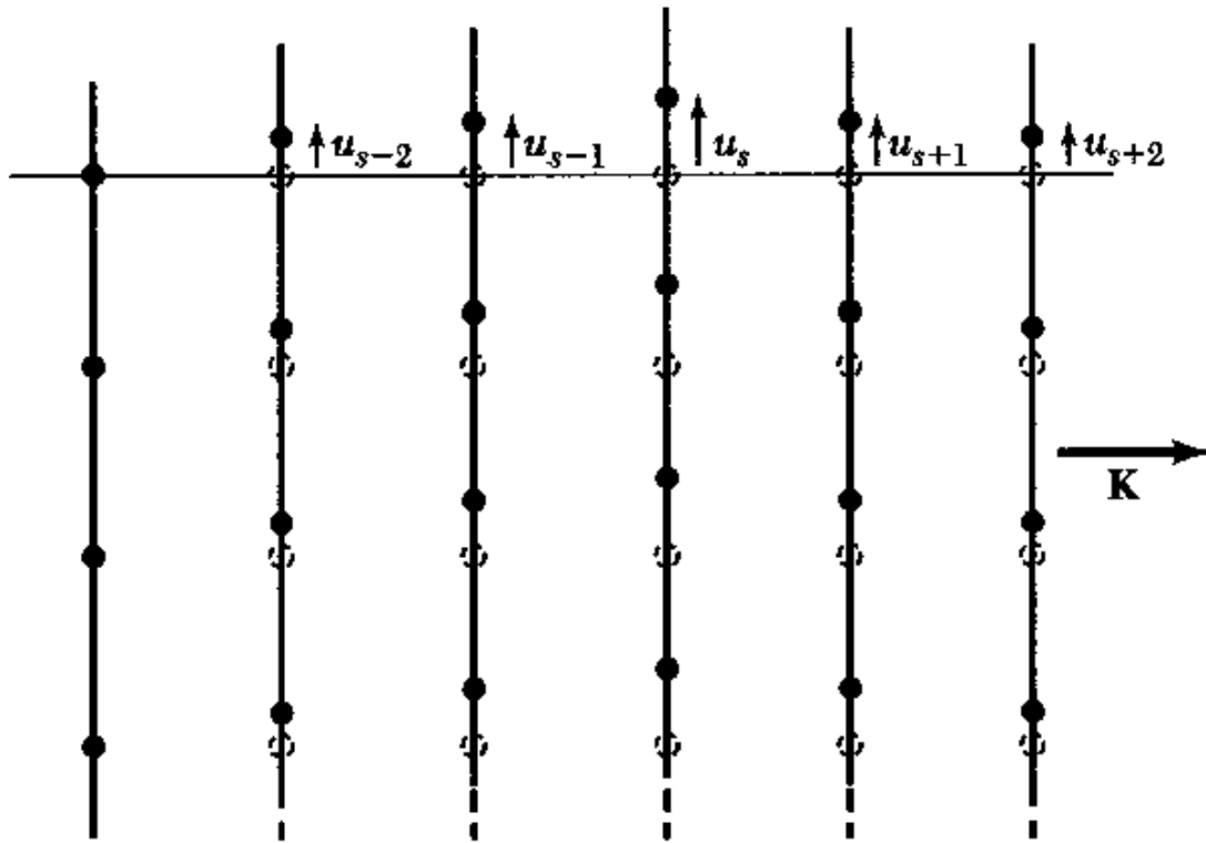
Modi trasversi
