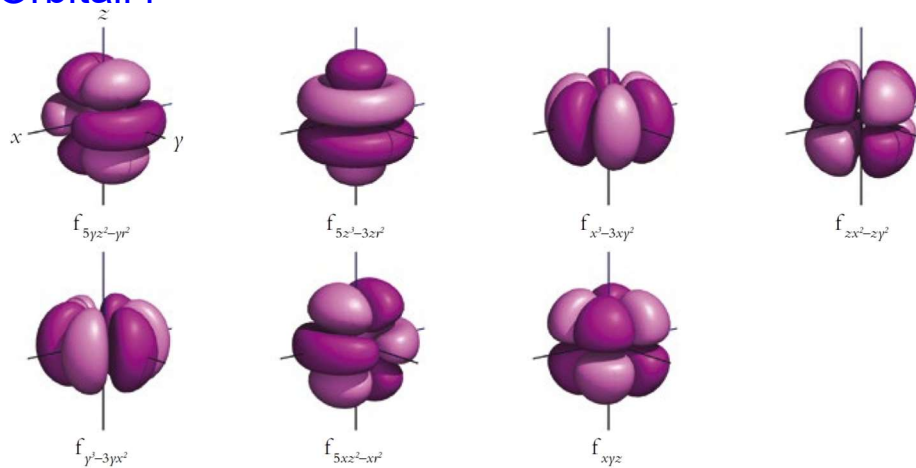
Figura 1D.11 I sette orbitali f di un guscio ( l = 3 ) hanno aspetto molto complesso, e nel testo non ne riproporremo la forma specifica; però la loro esistenza è importante per capire la tavola periodica, la presenza dei lantanoidi e degli attinoidi (i «lantanidi» e gli «attinidi») e le proprietà degli ultimi elementi del blocco d . Le sfumature più scure e più chiare indicano i diversi segni della funzione d'onda.
