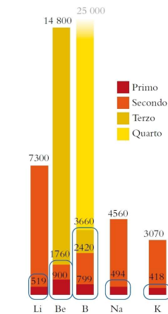
Figura 1F.10 I valori di energia relativi alle ionizzazioni successive per alcuni elementi dei gruppi principali. Si noti il grande aumento di energia necessario per allontanare un elettrone da un guscio interno. In ogni caso, le linee blu indicano la ionizzazione dal guscio di valenza.
