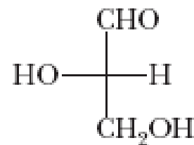
L-Gliceraldeide
