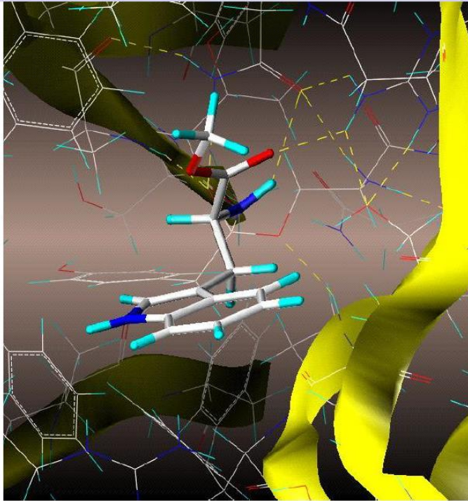
S-triptofano
