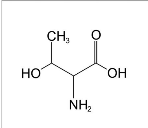
acido 2-ammino-3-idrossibutanoico
