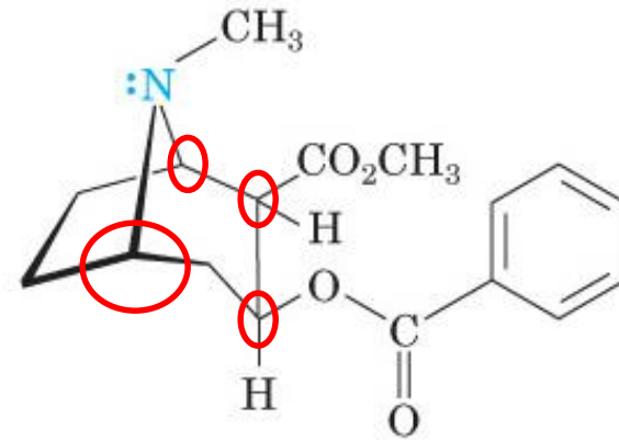
Cocaina
