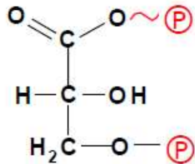
1,3 Bisfosfoglicerato
