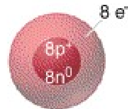
Ossigeno-16
