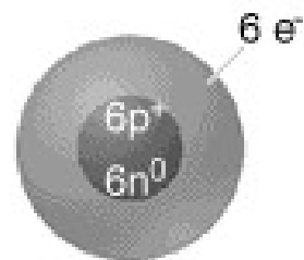
Carbonio-12
