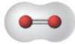
O 2
