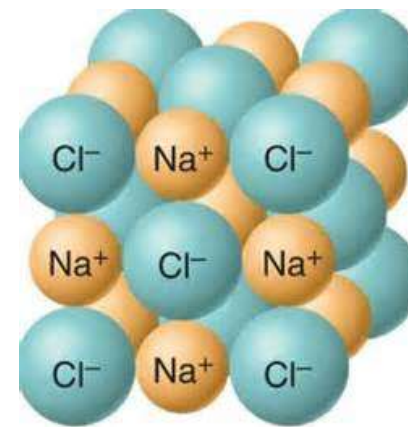
NaCl crystal
