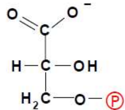
3 Fosfoglicerato
