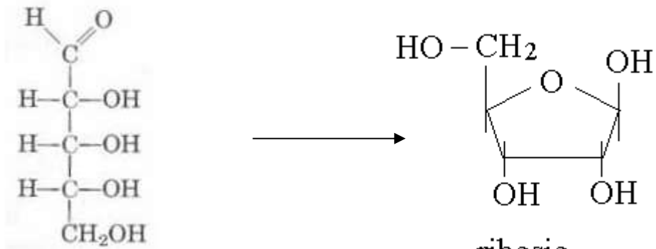
ribosio
