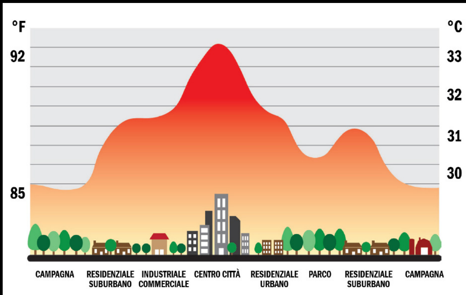
Rappresentazione grafica dell'isola di calore urbano.
