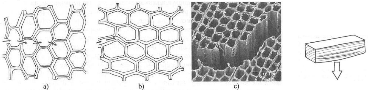
Figura 1.31 Modalità di rottura a livello anatomico del legno per trazione ortogonale alla fibratura: a) frattura delle pareti cellulari; b) frattura per delaminazione tra fibre adiacenti;
