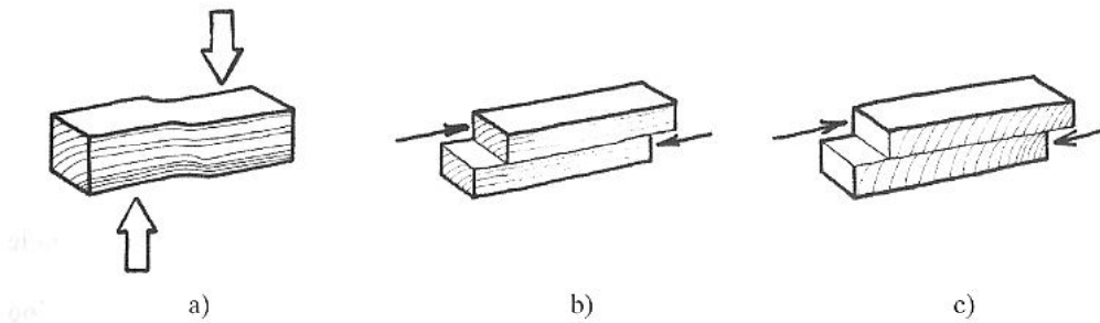
Figura 1.33 Proprietà meccaniche del legno sottoposto a taglio: a) nel taglio perpendicolare tendono a deformarsi le cellule perpendicolarmente al loro asse; b) nel taglio longitudinale si ha lo slittamento di cellule adiacenti longitudinalmente al loro asse; c) nel “rolling shear” le cellule tendono a separarsi ruotando una sull'altra.
