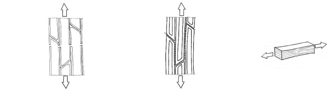
Figura 1.30 Modalità di rottura del legno, a livello anatomico, per trazione parallela alla fibratura.
