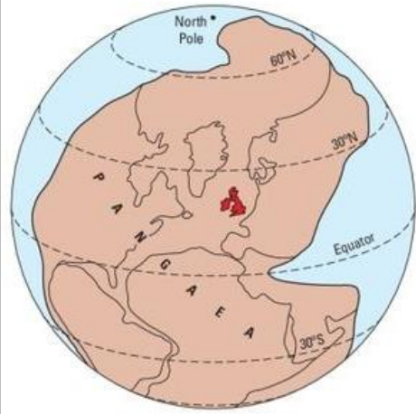
e) Permian–Triassic c. 250 Ma
