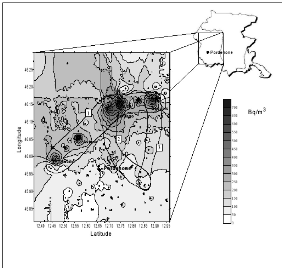
Figura 4.2.4 Distribuzione della concentrazione di radon negli edifici scolastici della provincia di Pordenone
