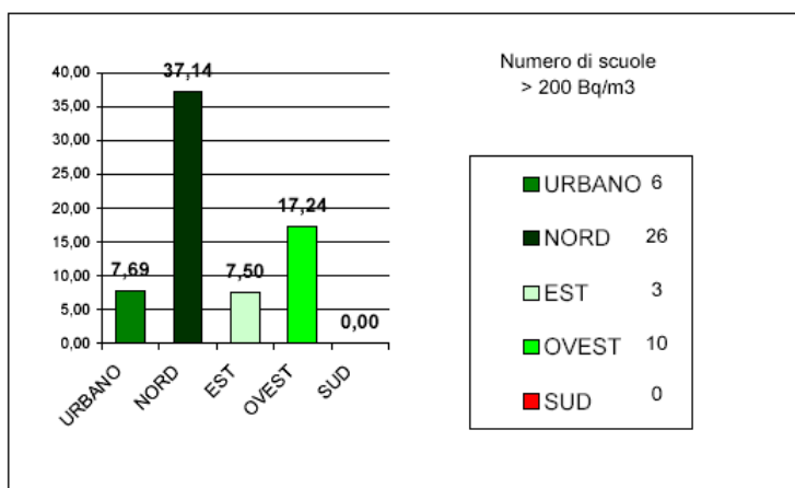
Figura 4.2.1 Percentuale (rispetto al totale del singolo distretto) e numero di scuole con medie superiori a 200 Bq/m 3
