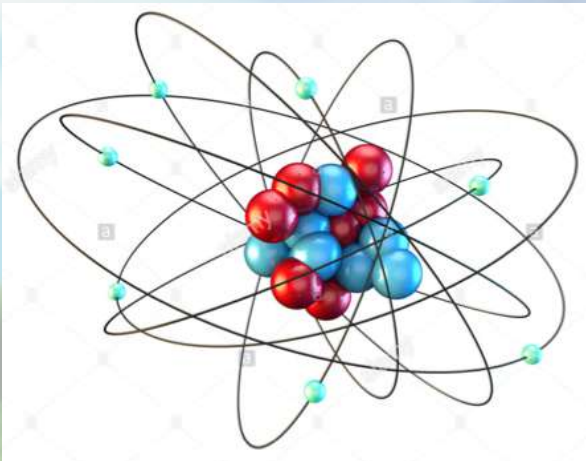
Atomo di Azoto
