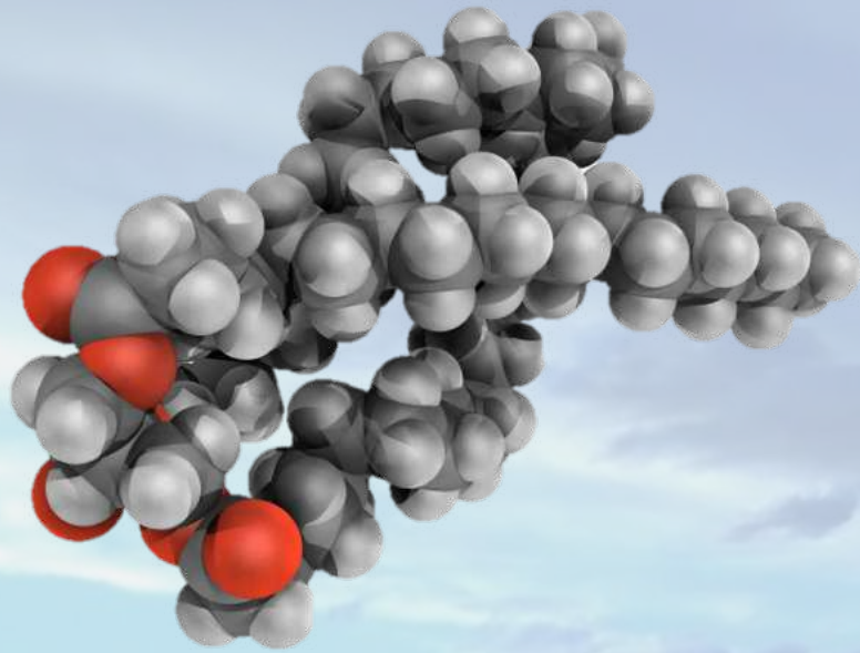
Trigliceridi
