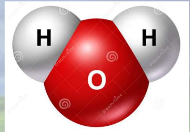
Molecola d'acqua
