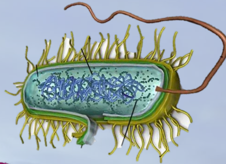
Procariote
