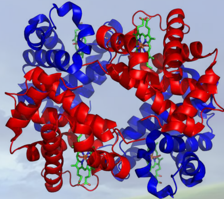
Emoglobina
