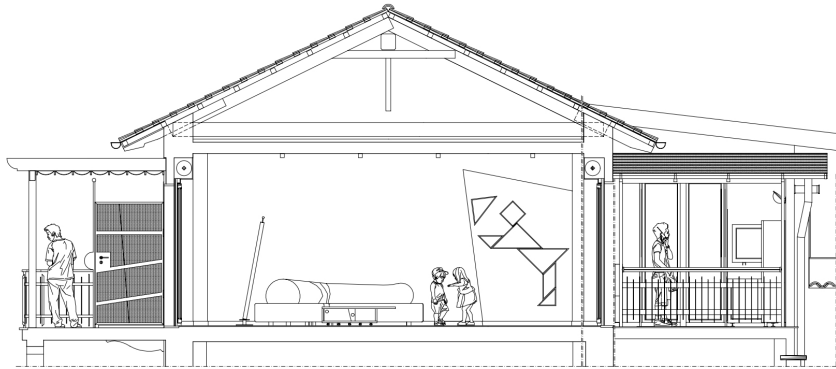
SEZIONE A-A
