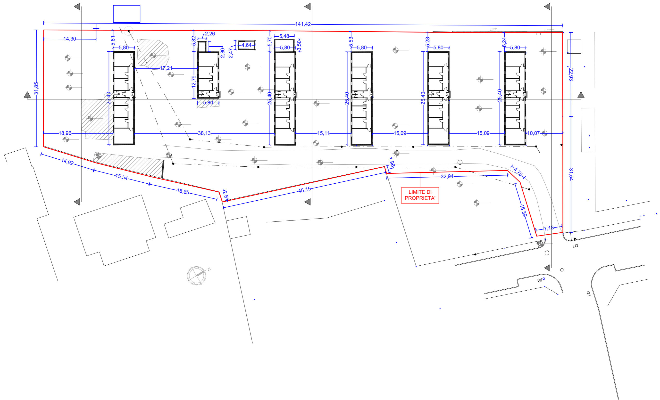
A3 - bordi e margini - scala 1:500
