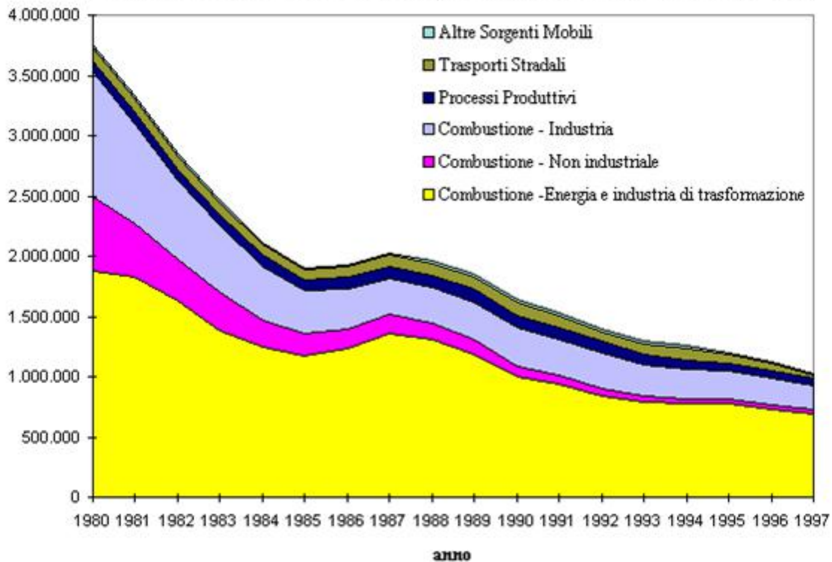
Emissioni nazionali di ossidi di zolfo (SO x ) in Italia per macrosettore 1980-1997 (ton.)
