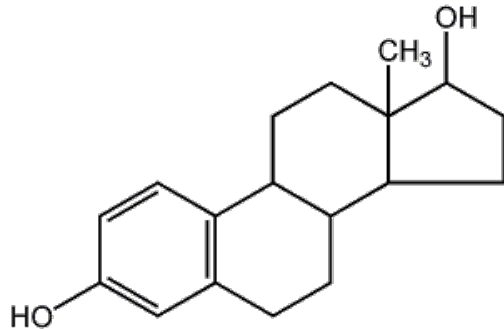
17- \beta -estradiolo
