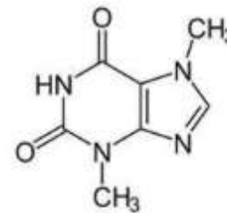
TEOBROMINA
