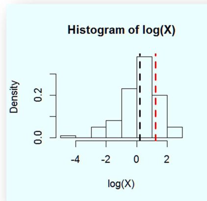
Figura 2 In nero: media di \log(X) ; in rosso: G.
