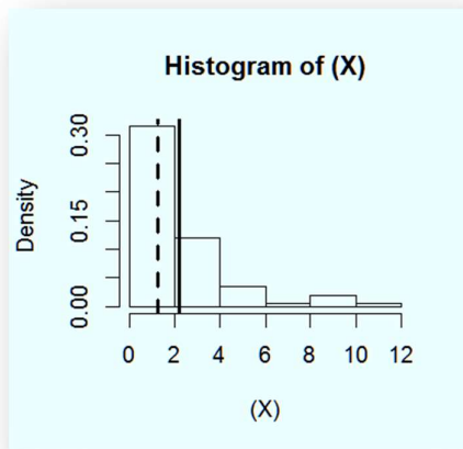
Figura 1. Linea continua: Media aritmetica. Linea tratteggiata: G.
