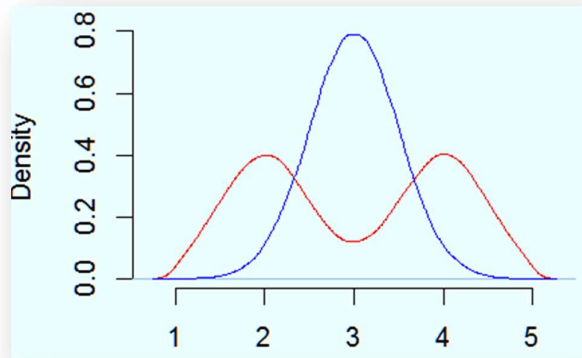
Figura 3 In rosso: bimodale (simmetrica); In blu: unimodale (simmetrica).
