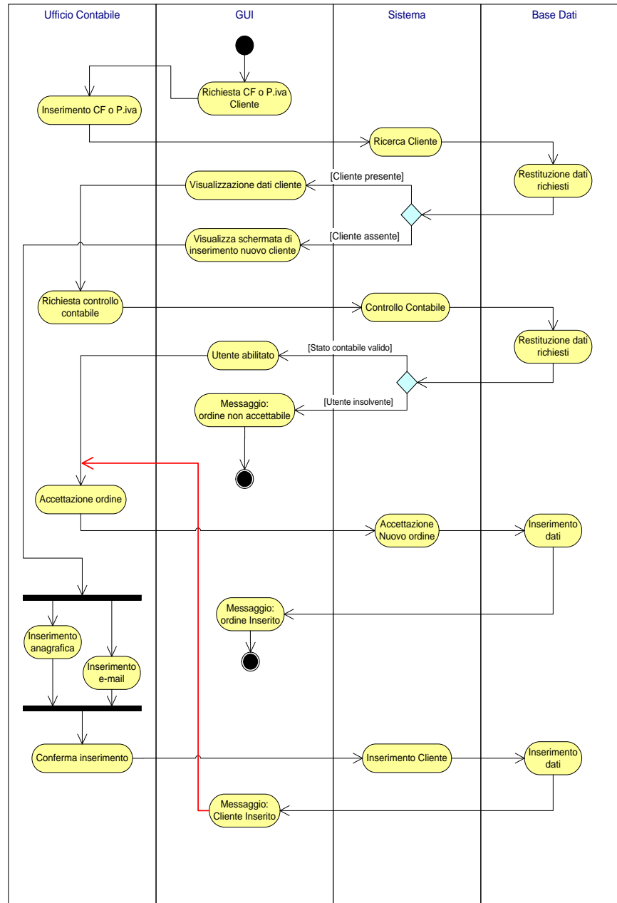
Activity Diagram - Use Case Accettazione Ordini
