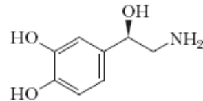
(R)-Norepinefrina
