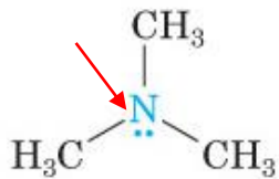
Trimetilammina
