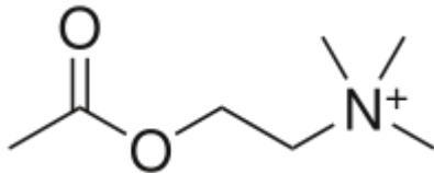
acetilcolina
