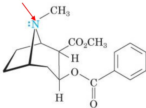
Cocaina
