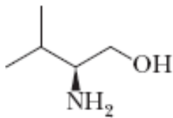
(S)-2-Ammino-3-metil-1-butanolo
