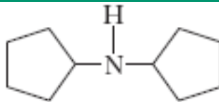
Diciclopentilammina
