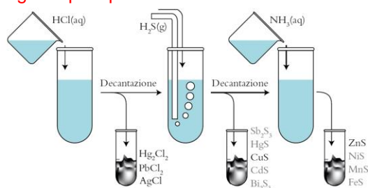
Figura 6J.4 Parte di un semplice schema di analisi qualitativa applicato per separare alcuni cationi. In un primo momento si separano tre cationi sotto forma di cloruri insolubili. In un secondo tempo si eliminano i cationi che formano solfuri insolubili facendoli precipitare a pH basso; infine i cationi residui sono fatti precipitare come solfuri, ma a pH più alto.
