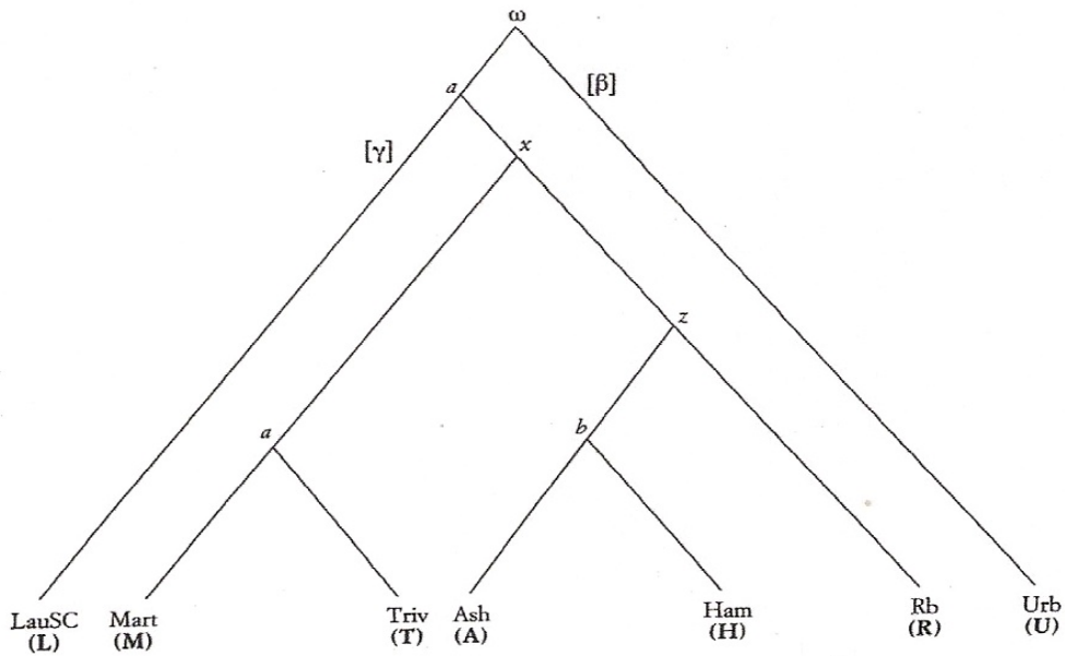
4. Stemma Inglese (2007).
