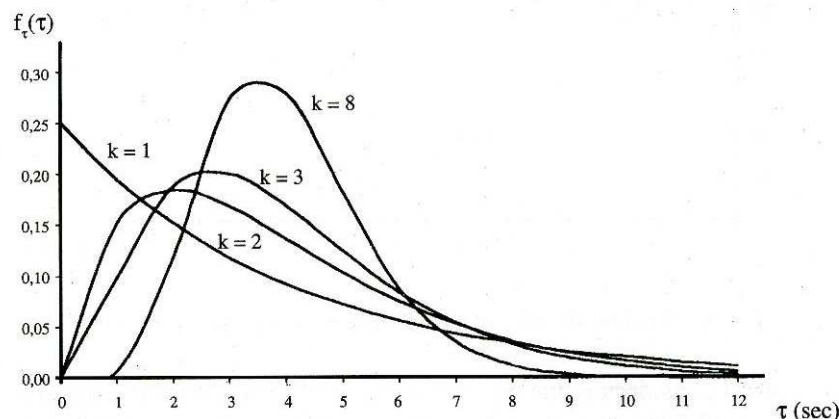
Fig.17b - Funzione densità di probabilità di Erlang per alcuni valori di k e con media costante \mu_{\tau} = k/\lambda = 4 sec
