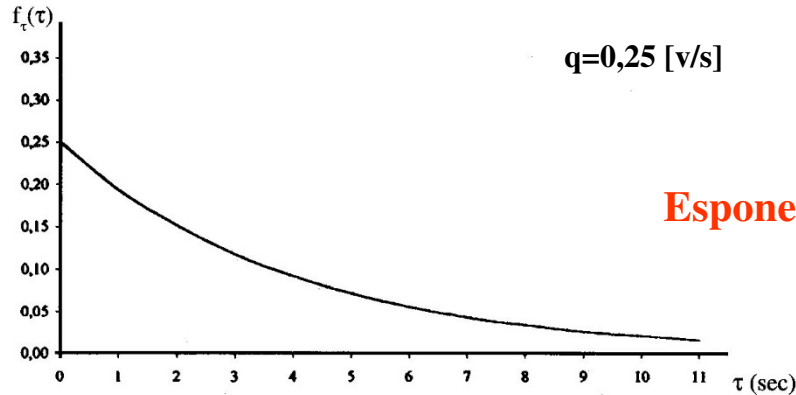
Fig.15 – Funzione densità di probabilità Esponenziale Negativa
