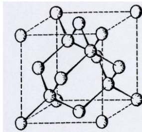
Fig. 12.2 Struttura del diamante. Ciascun atomo di carbonio ne coordina tetraedricamente altri quattro, cui è collegato da legami sp^3 ; i collegamenti vertice a vertice fra un numero indefinito di tetraedri determinano il formarsi di un'unica macromolecola grande quanto tutto il cristallo.
