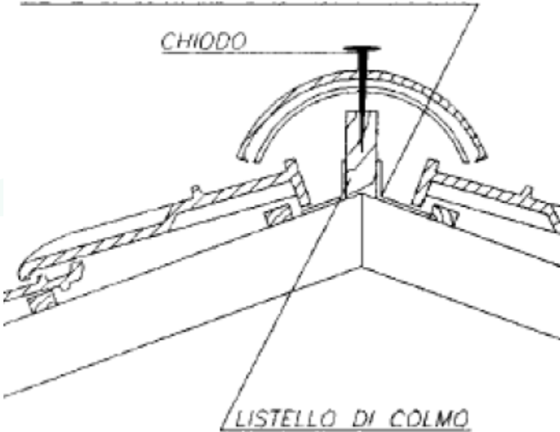
ELEMENTI METALLICI PER IL FISSAGGIO DEL LISTELLO DI COLMO
