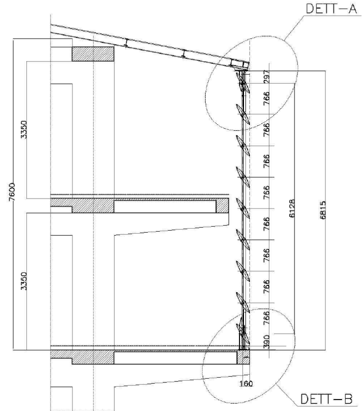
SEZIONE TIPO
