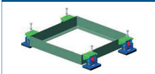
Figura 20 Basamento per ospitare una macchina da isolare
