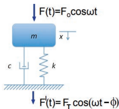
Figura 16 Effetto di una forza esterna su un sistema vibrante 'macchina semplice'
