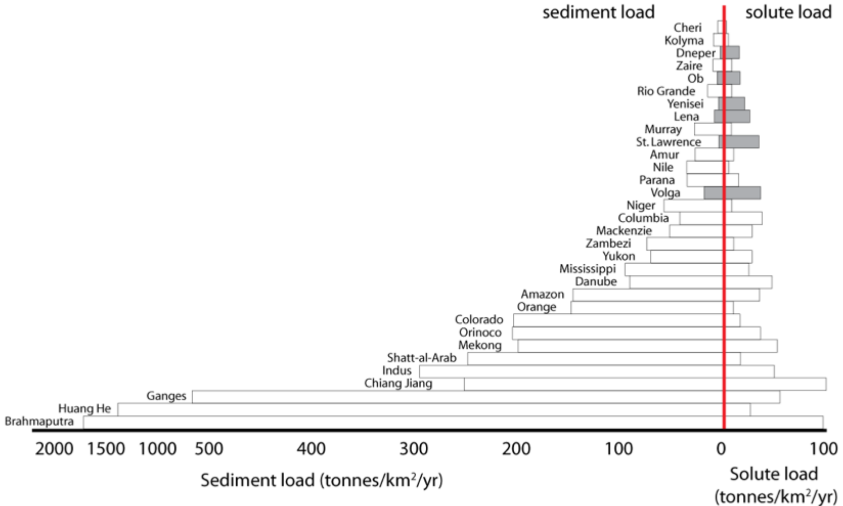
Carico sedimentario e di materiali sciolti dei principali fiumi nel mondo (Summerfield, 1991)
