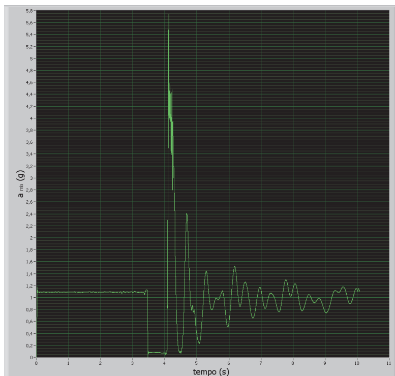
Figura A-55: Prova 80/2 F andamento di a_{mis} (g) rispetto al tempo [s]
