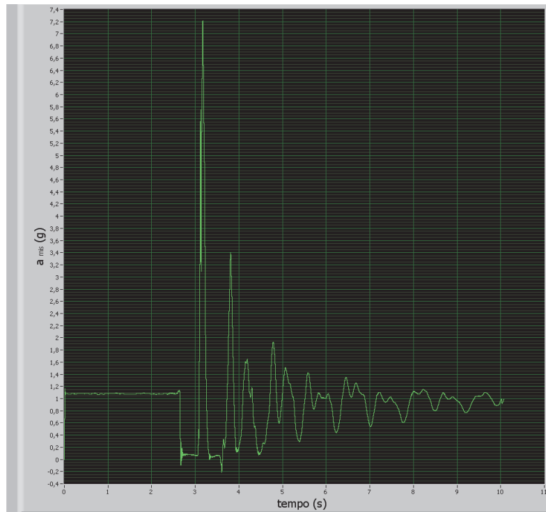
Figura A-1: Prova 60/1 F andamento di a_{mis} (g) rispetto al tempo [s]
