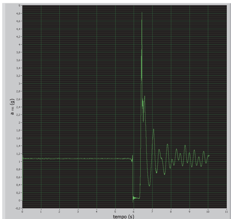
Figura A-287: Prova 120/1 I andamento di a_{mis} (g) rispetto al tempo [s]
