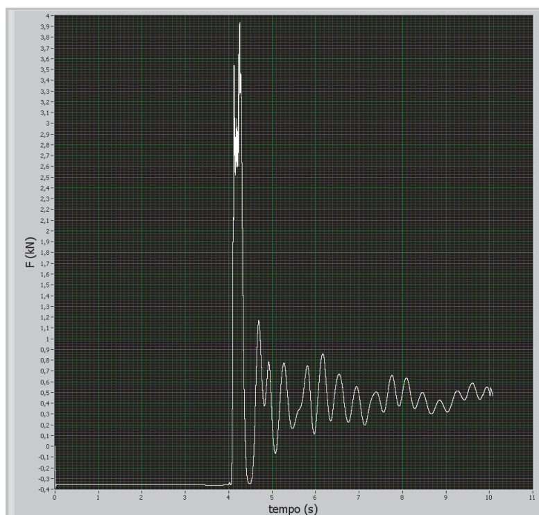
Figura A-56: Prova 80/2 F andamento di F [kN] rispetto al tempo [s]
