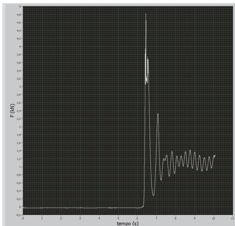
Figura A-288: Prova 120/1 I andamento di F [kN] rispetto al tempo [s]
