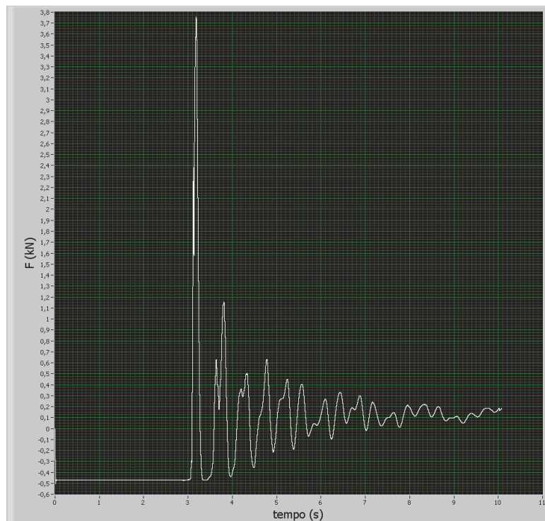
Figura A-2: Prova 60/1 F andamento di F [kN] rispetto al tempo [s]
